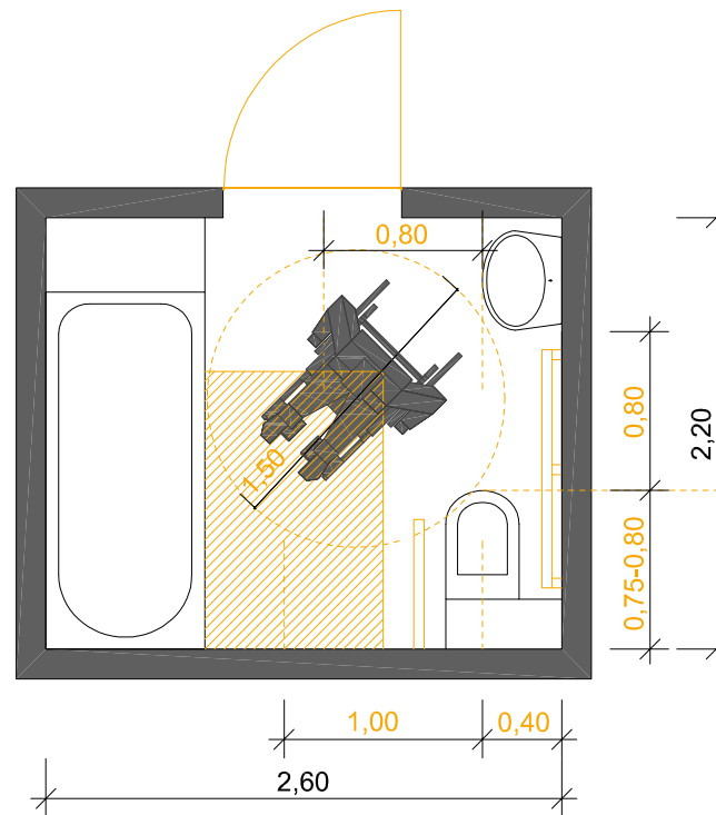
Badewanne - Vasca da bagno Tür lichte Breite 80cm - porta con luce netta 80cm
